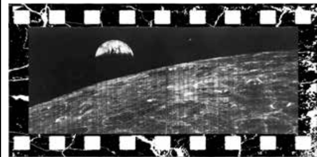
۱۱. اولین عکس زمین که از ماه گرفته شده
